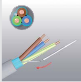
Bild 2: Schirmbeidraht (SB), mit transparentem Isolierschlauch versehen (elektrisch isolieren)
