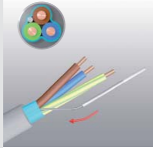
Bild 2: Schirmbeidraht (SB), mit transparentem Isolierschlauch versehen (elektrisch isolieren)
